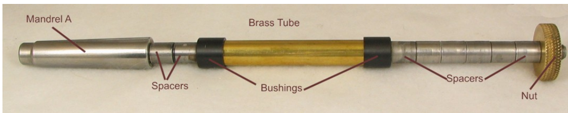
Mandrel Setup
