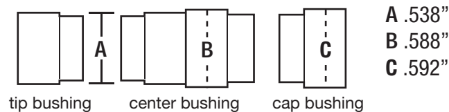
DIAGRAM D • PKOLBU
